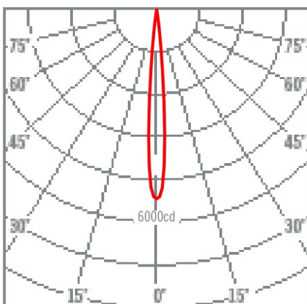
POLARDIAGRAM 10°:
