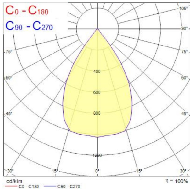
POLARDIAGRAM
