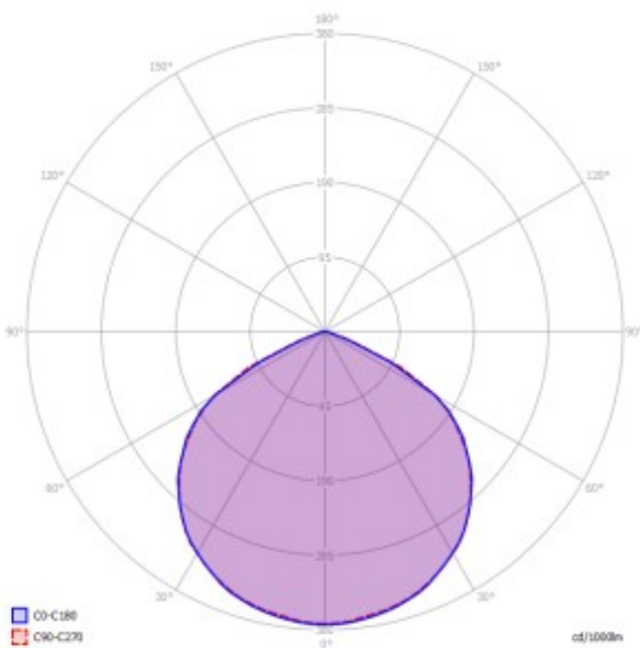
POLARDIAGRAM
