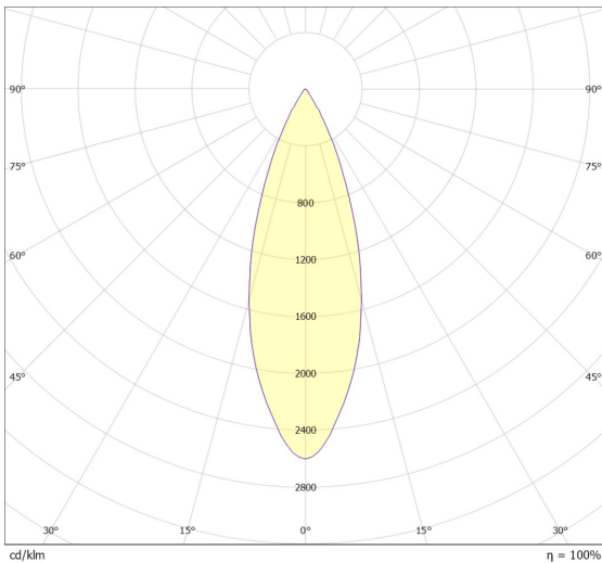
POLARDIAGRAM 24452—36°
