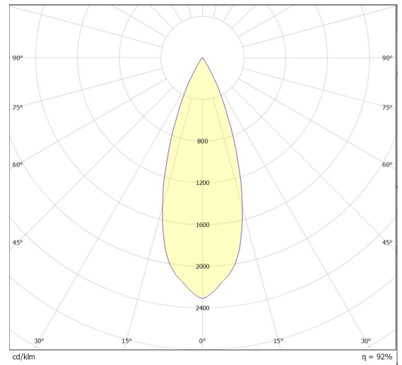
POLARDIAGRAM 24446—36°
