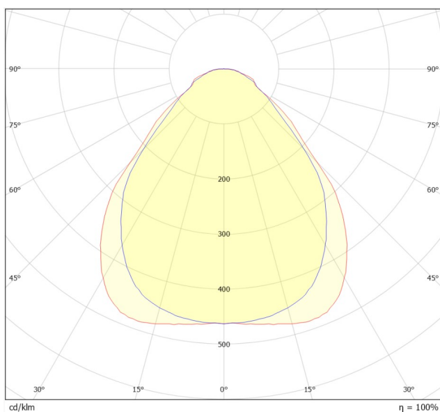
POLARDIAGRAM
