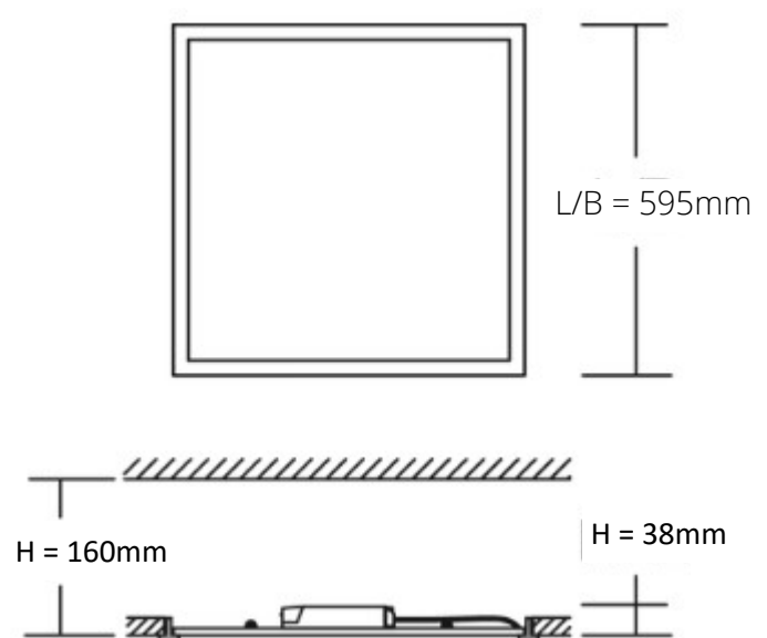
MÅLSKISSE
